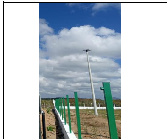
LUMINÁRIA 4 PÉTALAS EM POSTE DE CONCRETO CIRCULAR H=12M, ALTURA LIVRE 10,20M, LÂMPADA VAPOR METÁLICO DE 400W, INCLUSIVE O POSTE
